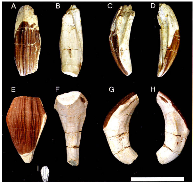
Fig.2 Lanzhousaurus magnidens gen. et sp. nov.
